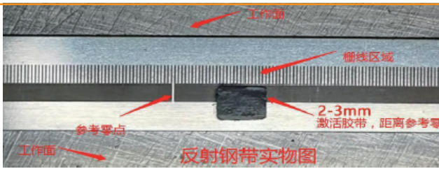
图 3: 反射钢带实物图
