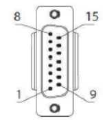
DB15针插头
